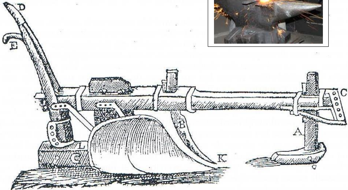
Reproductie van de houtgravure van een Kempense ploeg, waarschijnlijk daterend uit het midden van de achttiende eeuw, gepubliceerd in het boek van Isfridus Thijs, van 1792. Hij heeft een verstelbaar voetje en een ploegkam vooraan; achteraan één ploegstaart met een handvat, een holronde schaar die zonder onderbreking de welving van het raster voortzet, en een heugel.
